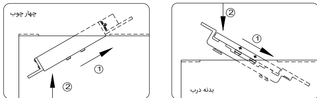
نصب بست‌های فلزی در صورت نیاز
