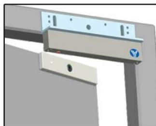
نصب براکت L شکل
