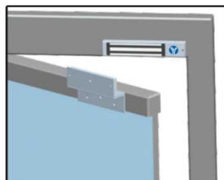
نصب براکت ZL شکل
